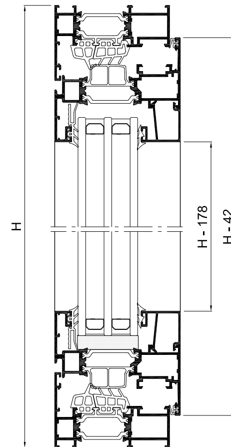
Sección B-B'
