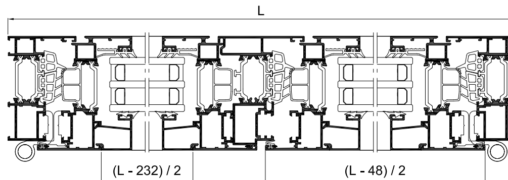
Sección A-A'
